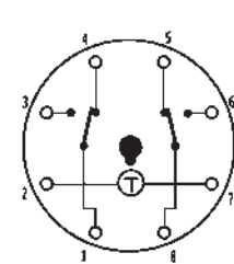
TERMINAL WIRING
