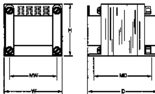
Fig. B Solder Lugs
