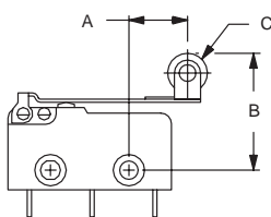
FIG. 1 Lever Roller
