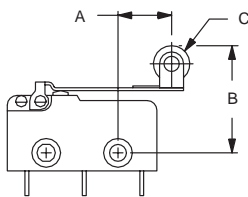
FIG. 2 Lever Roller
