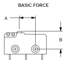
FIG. 7 Pin Plunger
