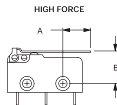
FIG. 3 Lever
