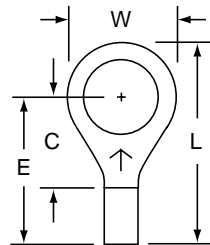
M14-516R/S Stud Size: 5/16 Wire Range: 16-14
