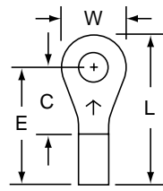
M14-6R/L Stud Size: 6 Wire Range: 16-14
