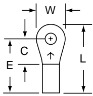
M14-2R/S Stud Size: 2 Wire Range: 16-14
