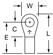
M14-6R/S Stud Size: 6 Wire Range: 16-14
