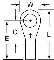
M14-10R/L Stud Size: 10 Wire Range: 16-14
