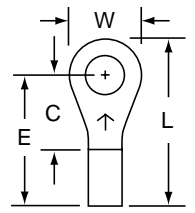
M14-8R/L Stud Size: 8 Wire Range: 16-14
