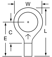
M14-38R Stud Size: 3/8 Wire Range: 16-14
