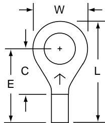
M14-14R/S Stud Size: 1/4 Wire Range: 16-14
