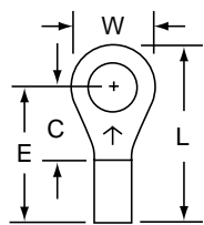
M14-10R Stud Size: 10 Wire Range: 16-14
