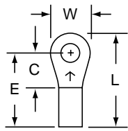
M14-4R/S Stud Size: 4 Wire Range: 16-14
