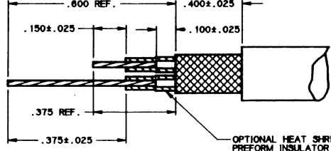
TWINAX STRIP \Delta (RAYTHEON MS-20084/1-001)
