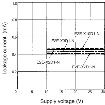
E2E-X□D□
