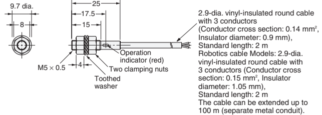
Fig. 4: E2E-X1
