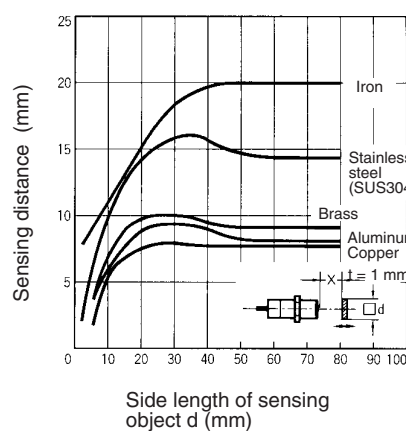
E2E-X20MD
