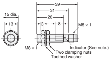
Fig. 28: E2E-X2D□-M3G/E2E-X1R5E□-M3/F□-M3
