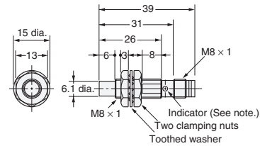
Fig. 29: E2E-X4MD□-M3G/E2E-X2ME□-M3/F□-M3
