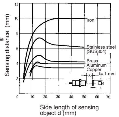
E2E2-X10D□
