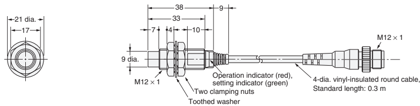
Fig. 32: E2E-X7D1-M1GJ E2E-X7D1-M1J-T
