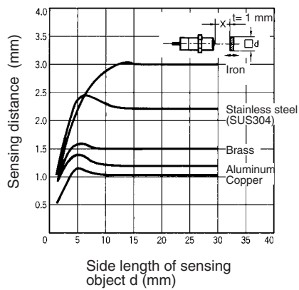
E2E2-X3D□
