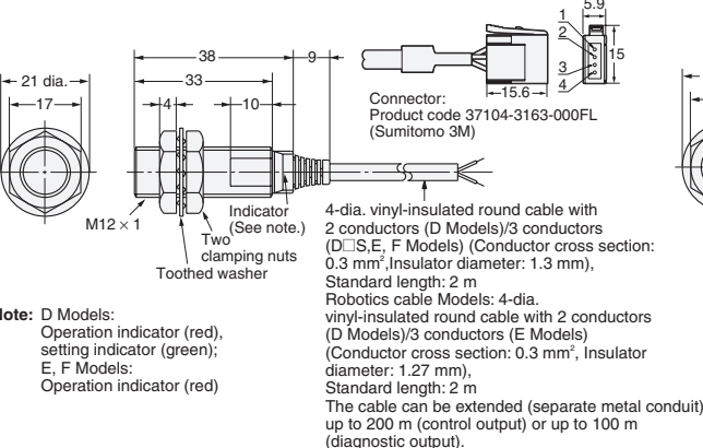
Fig. 9: E2E-X3D-N E2E-X2E/F
