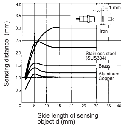
E2E-X4MD
