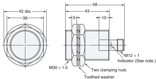
Fig. 26: E2E-X10D□-M1(G)/E2E-X10E□-M1/F□-M1 E2E-X10Y□-M1
