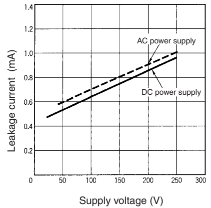
E2E-X□T1 DC/AC
