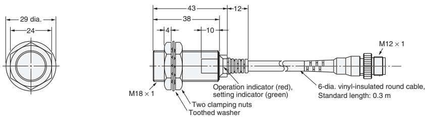
Fig. 32: E2E-X7D1-M1GJ E2E-X7D1-M1J-T
