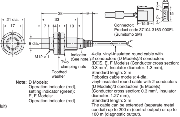
Fig. 10: E2E-X8MD E2E-X5ME/F
