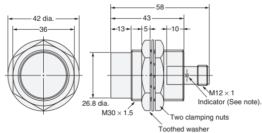
Fig. 27: E2E-X20MD□-M1(G)/E2E-X18ME□-M1/F□-M1 E2E-X18MY□-M1
