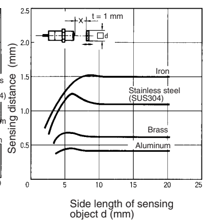
E2E-X1R5E / F E2E-X1R5Y
