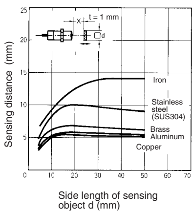
E2E-X14MD
