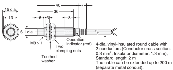
Fig. 10: E2E-X8MD E2E-X5ME/F
