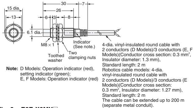
Fig. 8: E2E-X2MY
