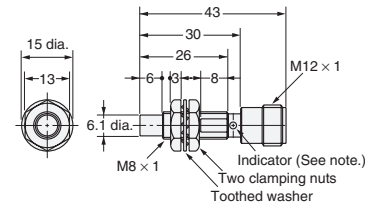
Fig. 19: E2E-X4MD□-M1(G) E2E-X2ME□-M1/F□-M1
