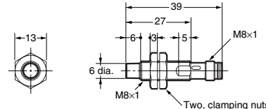
E2A-S08KN04-M5-□□
