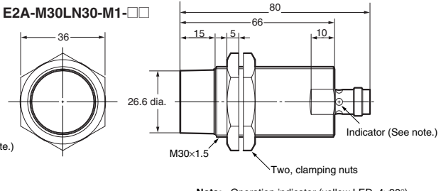
E2A-M30LN30-M1-□□
