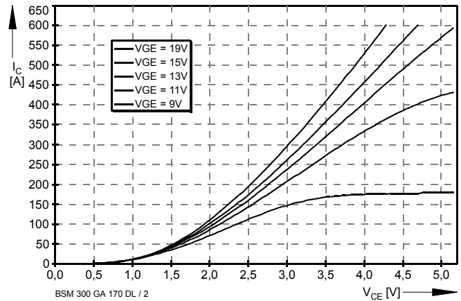
Bild / Fig. 2 Ausgangskennlinienfeld (typisch) / Output characteristic (typical) I_C = f(V_{CE}) T_{Ji} = 125^\circ\text{C}
