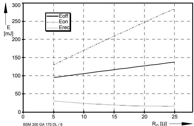
Bild / Fig. 6 Schaltverluste (typisch) / Switching losses (typical) E_{on} = f(R_G) , E_{off} = f(R_G) , E_{rec} = f(R_G) I_C = 300\text{A} , V_{CE} = 900\text{V} , T_J = 125^\circ\text{C}
