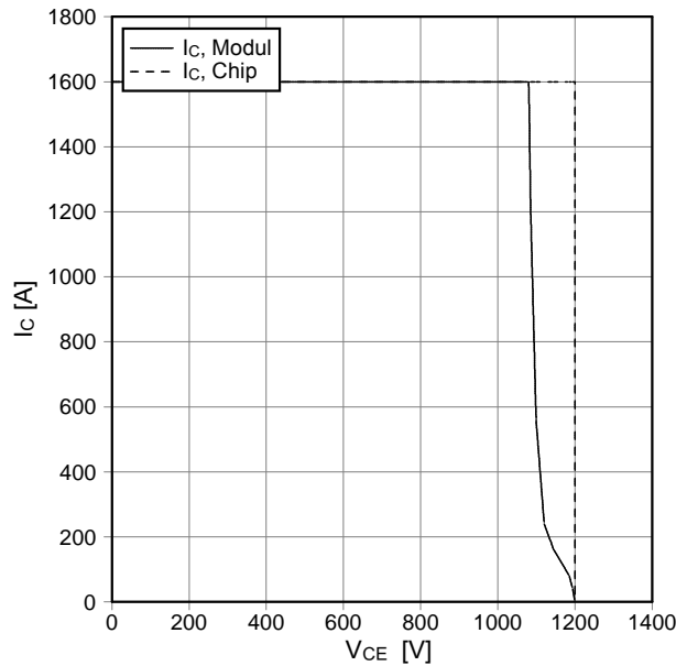
Sicherer Rückwärts-Arbeitsbereich IGBT-Wr. (RBSOA) reverse bias safe operating area IGBT-inv. (RBSOA) I_C = f(V_{CE}) V_{GE} = \pm 15 \text{ V} , R_{Goff} = 0.91 \text{ Ω} , T_{vj} = 125^\circ\text{C}
