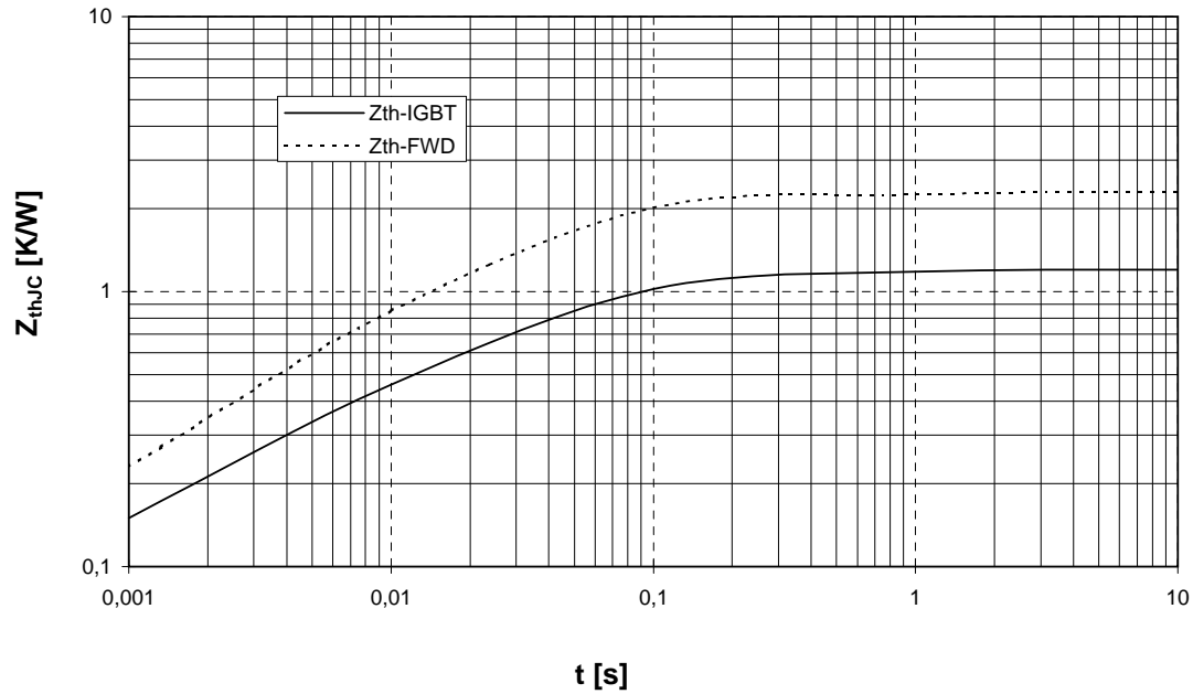
Transienter Wärmewiderstand Wechselr. Transient thermal impedance Inverter
