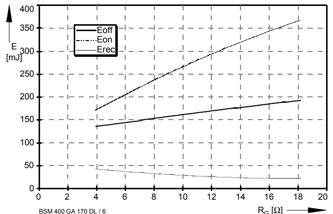
Bild / Fig. 6 Schaltverluste (typisch) / Switching losses (typical) E_{on} = f(R_C) , E_{off} = f(R_C) , E_{rec} = f(R_C) I_C = 400A , V_{CE} = 900V , T_j = 125^\circ C
