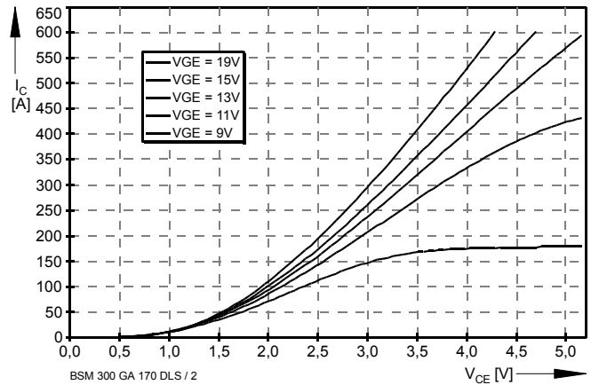
Bild / Fig. 2 Ausgangskennlinienfeld (typisch) / Output characteristic (typical) I_C = f(V_{CE}) T_{Ji} = 125^\circ C
