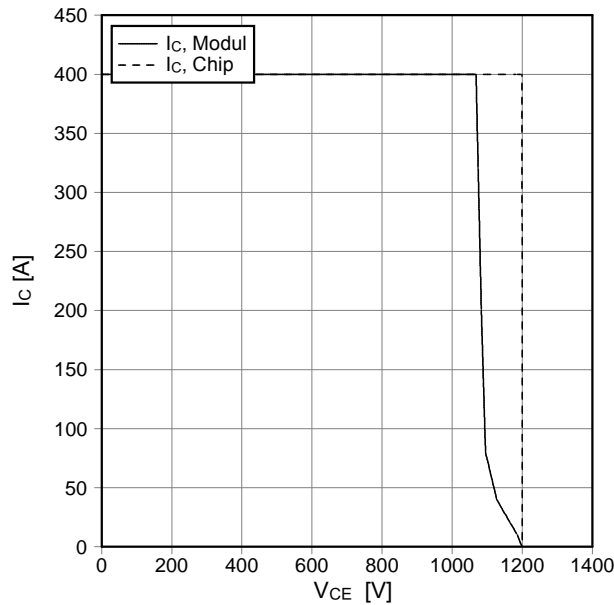
Sicherer Rückwärts-Arbeitsbereich IGBT-Wr. (RBSOA) reverse bias safe operating area IGBT-inv. (RBSOA) I_C = f(V_{CE}) V_{GE} = \pm 15\text{ V} , R_{Goff} = 3.6\ \Omega , T_{vj} = 125^\circ\text{C}
