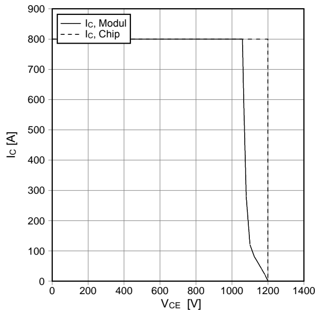
Sicherer Rückwärts-Arbeitsbereich IGBT-Brems-Chopper reverse bias safe operating area IGBT-brake-chopper I_C = f(V_{CE}) V_{GE} = \pm 15\text{ V} , R_{Goff} = 1.8\ \Omega , T_{vj} = 125^\circ\text{C}
