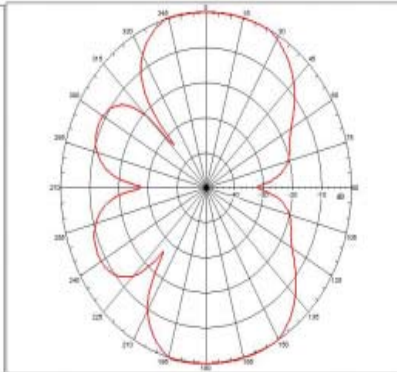
E-PLANE
