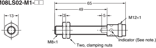
E2A-S08LS02-M1-□□ E2A-M08LS02-M1-□□
