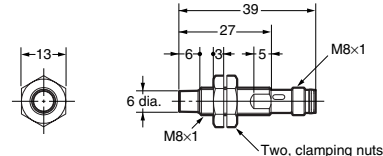
E2A-S08KN04-M5-□□
