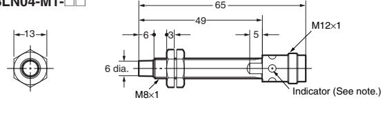
E2A-S08LN04-M1-□□ E2A-M08LN04-M1-□□
