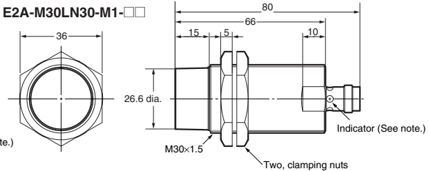
E2A-M30LN30-M1-□□
