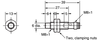
E2A-S08KN04-M5-□□
