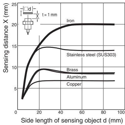
E2A-M30KN20
