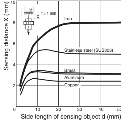
E2A-M12□N08
