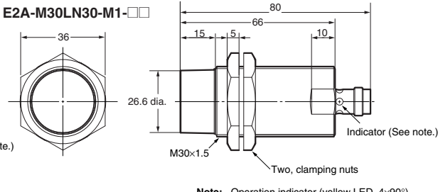
E2A-M30LN30-M1-□□
