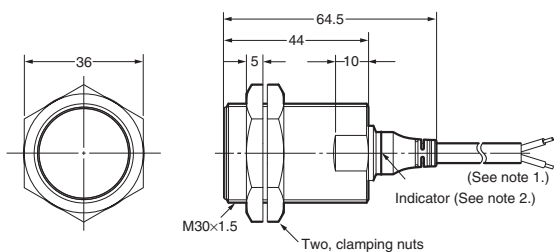
E2A-M30KS15-WP-□□
