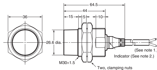
E2A-M30KN20-WP-□□
