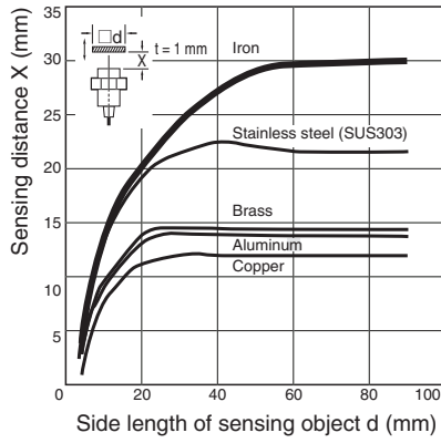
E2A-M30LN30
