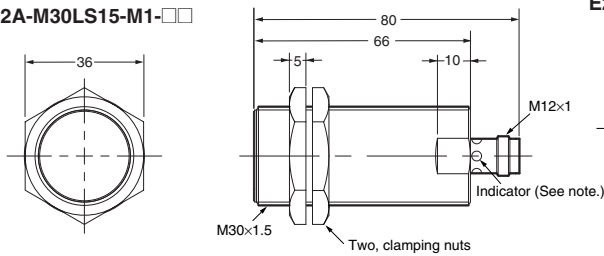
E2A-M30LS15-M1-□□
