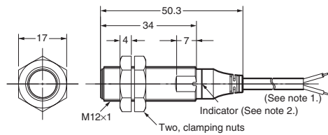
E2A-M12KS04-WP-□□
