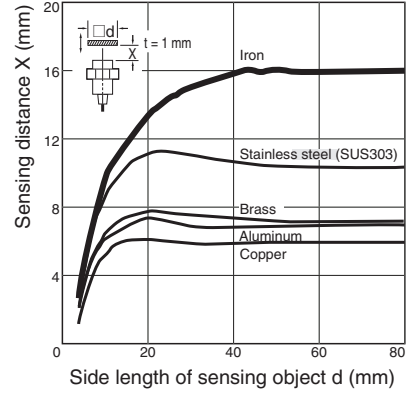
E2A-M18□N16
