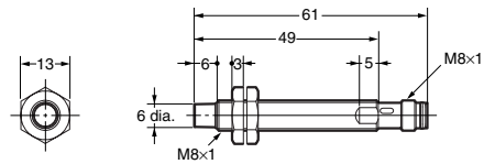
E2A-S08LN04-M5-□□
