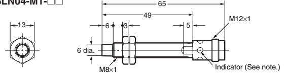
E2A-S08LN04-M1-□□ E2A-M08LN04-M1-□□
