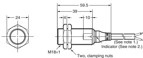
E2A-M18KS08-WP-□□
