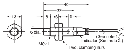
E2A-S08KN04-WP-□□
