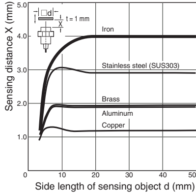
E2A-S08□N04/M08□N04
