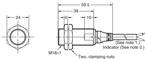
E2A-M18KS08-WP-□□
