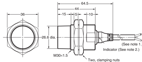
E2A-M30KN20-WP-□□
