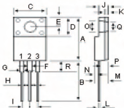
Dimensions : Millimetres
