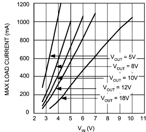
20059148 Max. Load Current (typ) vs VIN - "X"
