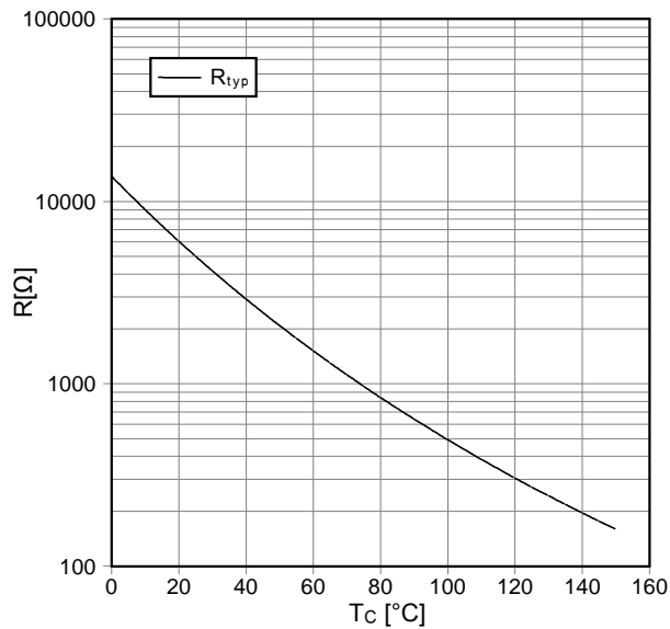
NTC-Temperaturkennlinie (typisch) NTC-temperature characteristic (typical) R = f(T)
