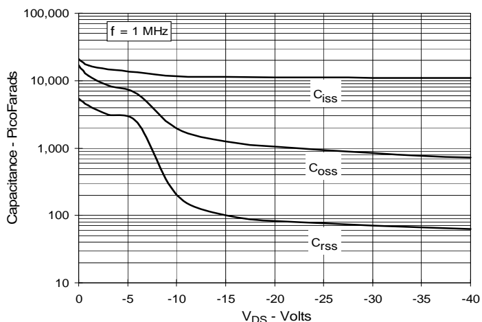
Fig. 11. Capacitance
