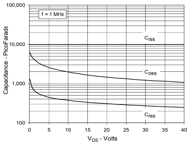
Fig. 11. Capacitance
