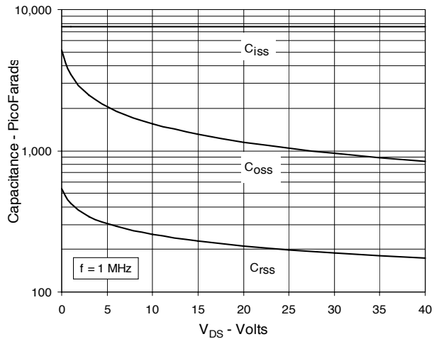
Fig. 11. Capacitance
