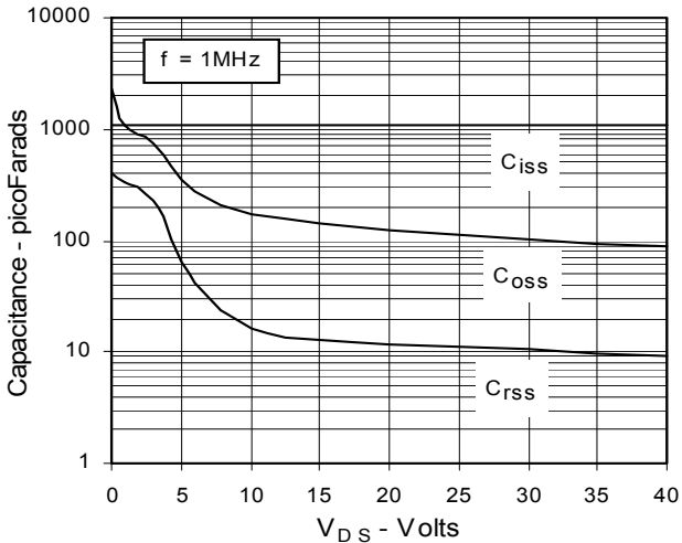
Fig. 11. Capacitance
