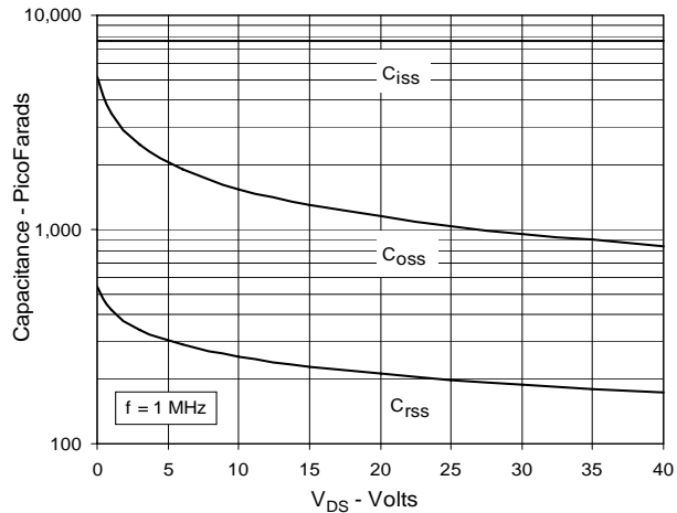
Fig. 11. Capacitance
