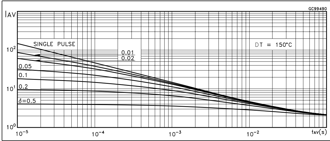
Figure 18. Allowable I AV vs. time in avalanche
