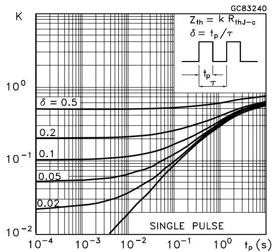
Thermal Impedance
