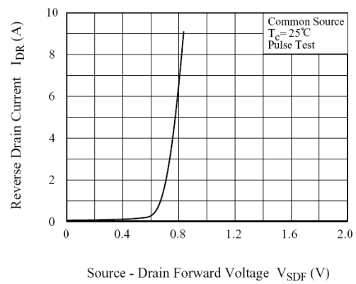
Fig6. I_{DR} - V_{SDF}
