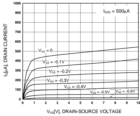
Figure 2. I_D - V_{DS}
