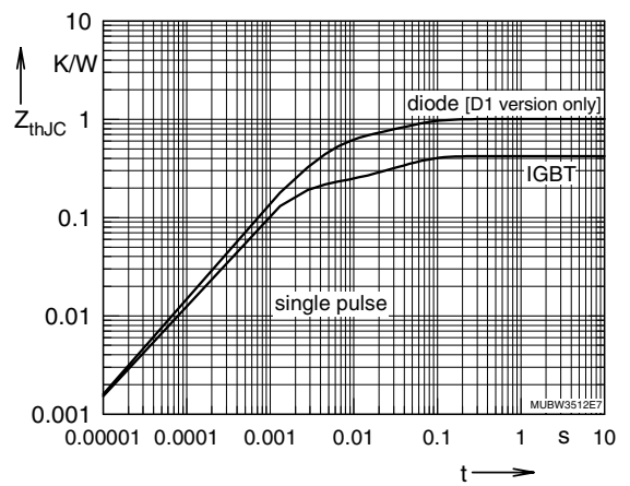
Fig. 6 Typ. transient thermal impedance
