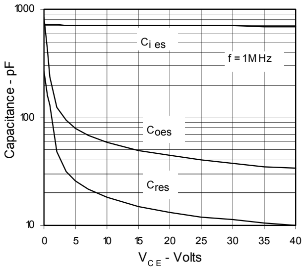
Fig. 12. Capacitance
