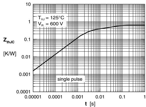
Fig. 10 Typ. transient thermal impedance
