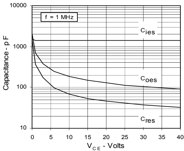
Fig. 15. Capacitance
