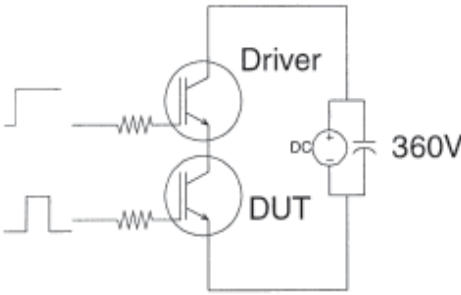
Fig.C.T.3 - S.C.SOA Circuit
