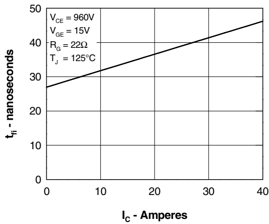
Fig. 7 Typ. Fall Time
