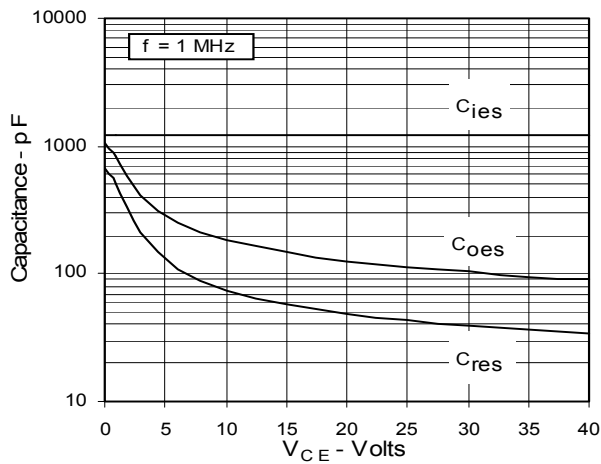
Fig. 15. Capacitance
