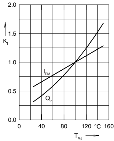
Fig. 21. Dynamic parameters Q_r , I_{RM}
