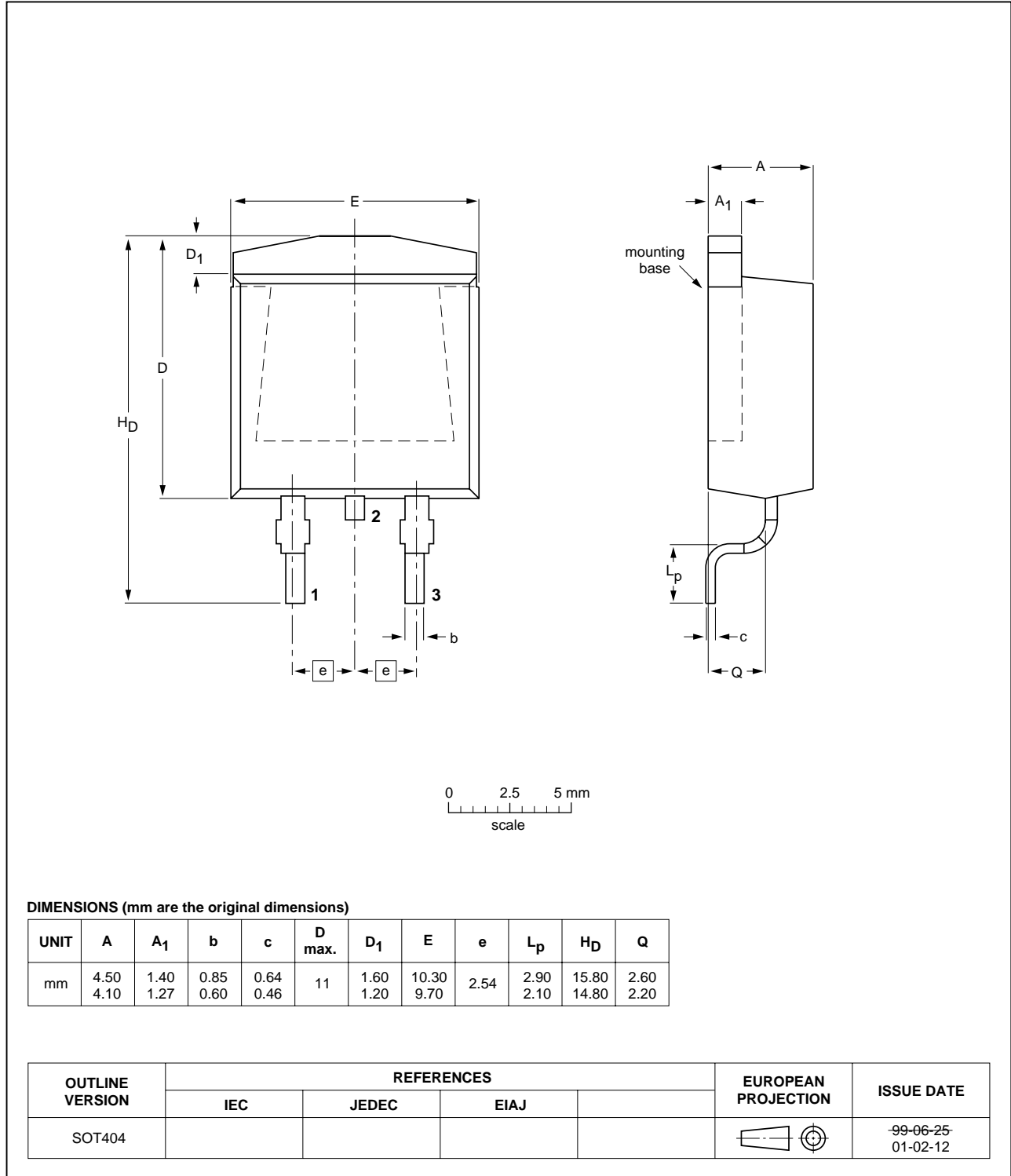
Fig 9. SOT404 (D 2 -PAK).
