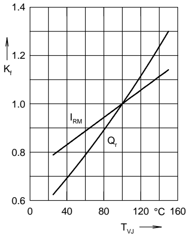
Fig. 4 Dynamic parameters Q_r , I_{RM}
