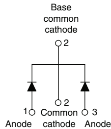
D²PAK
