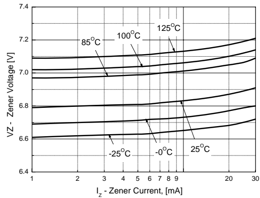
Figure 4. MM3Z6V8C Zener current vs. Zener Voltage
