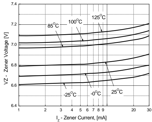
Figure 4. MM3Z6V8C Zener current vs. Zener Voltage
