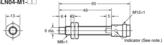
E2A-S08LN04-M1-□□ E2A-M08LN04-M1-□□
