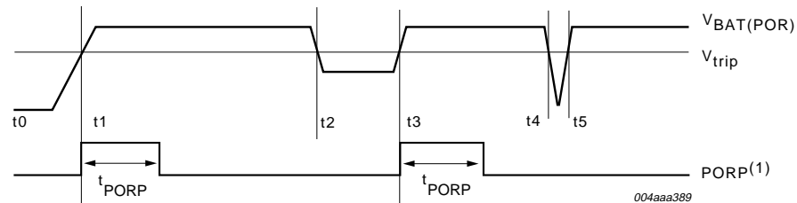
Fig 33. Internal POR timing.
