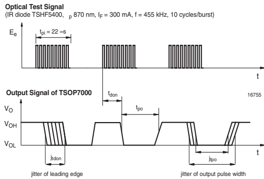
Figure 2. Output Function (mit Jitter)
