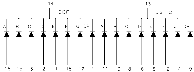
F.LTC-5753X-01
