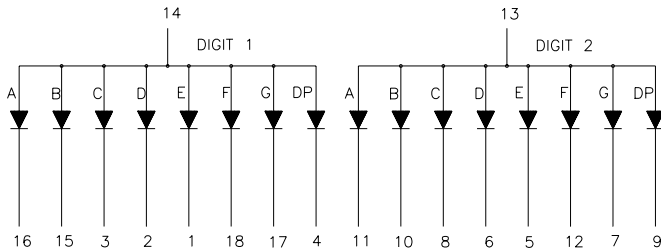
E.LTC-5653X-01
