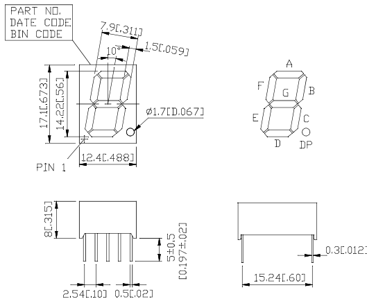
A. LTS-5X01A/5X03A
