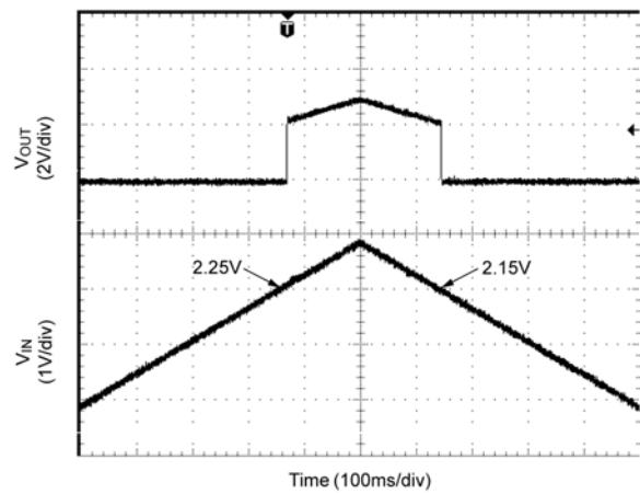
UVLO
