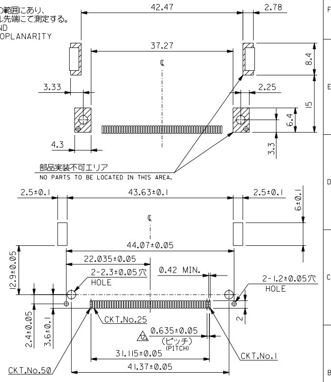
基板推奨寸法 RECOMMENDED P.C.B. LAYOUT
