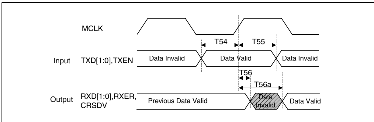
Figure 22. RMIITiming Parameters
