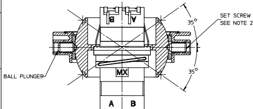
SECTION A-A SCALE 2.5:1
